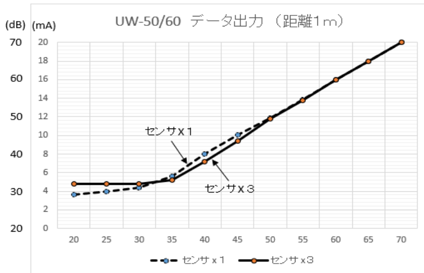
第3図 データ出力特性
