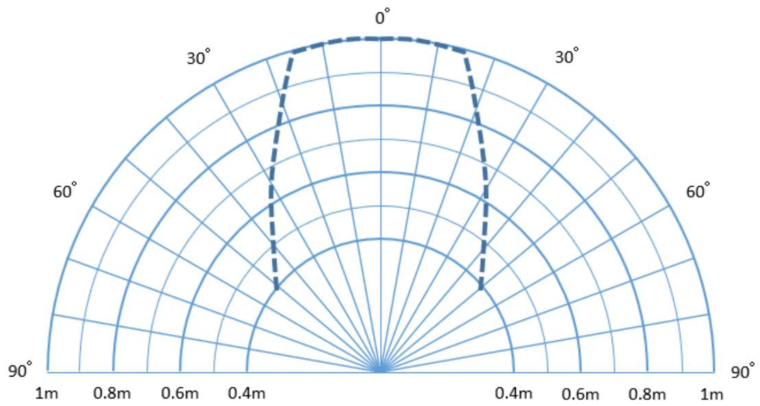
第6図 センサーカバー範囲
